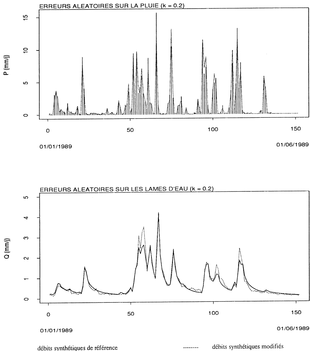
Fig. 6.2 - Débits synthétiques de référence et débits synthétiques modifiés par des erreurs aléatoires ( k = 0,2 )
