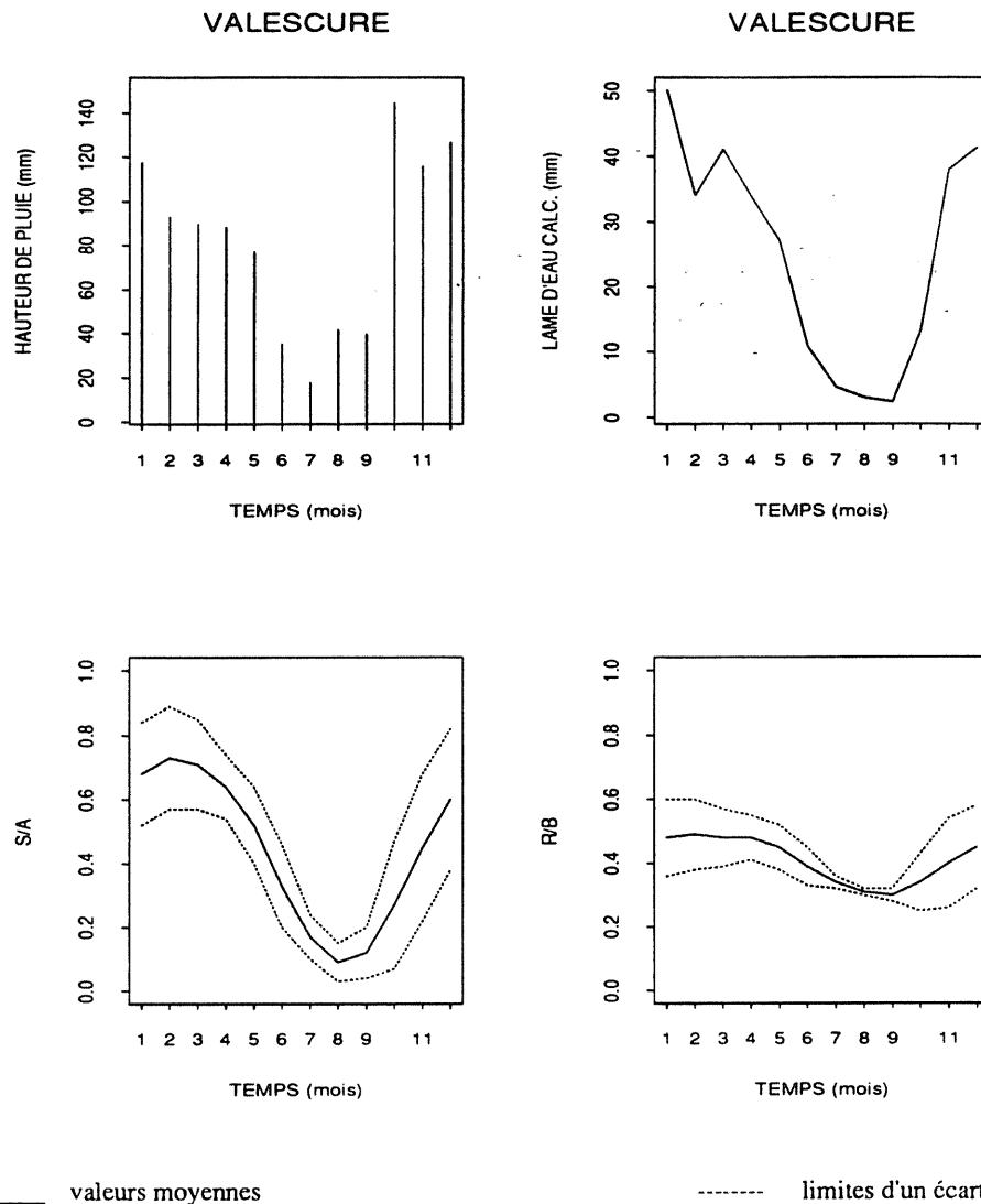
Fig. 3.12 b - Valeurs moyennes mensuelles de P , de Q_{calc} , de S/A et de R/B . Valescure au Bourdins calage : 1981-1989
