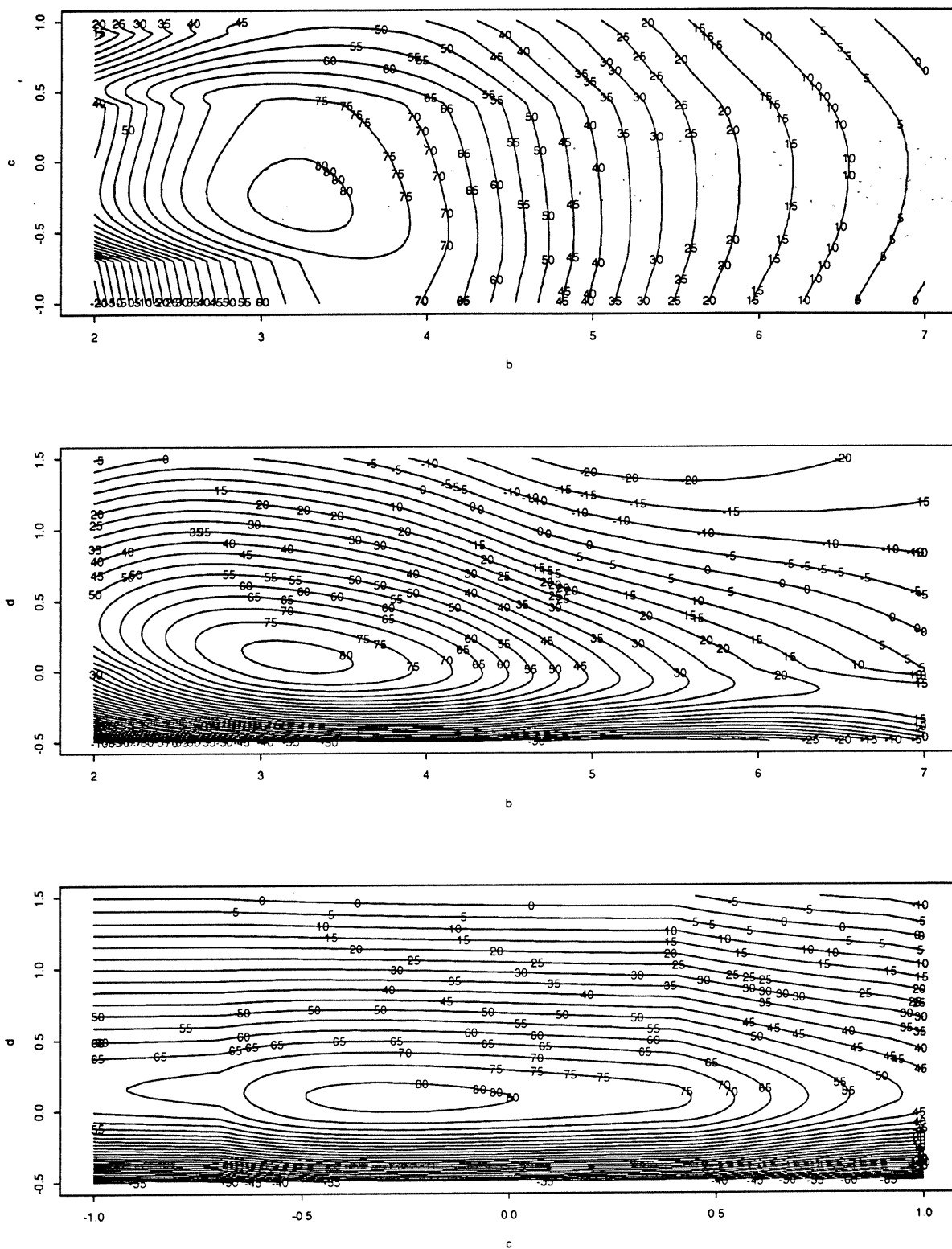
Fig. 5.21 - Méthode EG appliquée au modèle GR4J - courbes d'isocritère paramètres a-b , a-c , a-d , b-c , b-d et c-d - fonction critère (critère de NASH) Bassin versant de l'Orgeval pour la période 1975-1977
