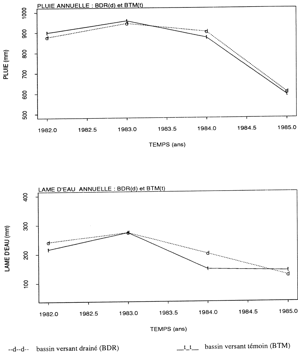
Fig. 7.4 - Bassins versants BTM et BDR - Précipitations et lames d'eau annuelles
