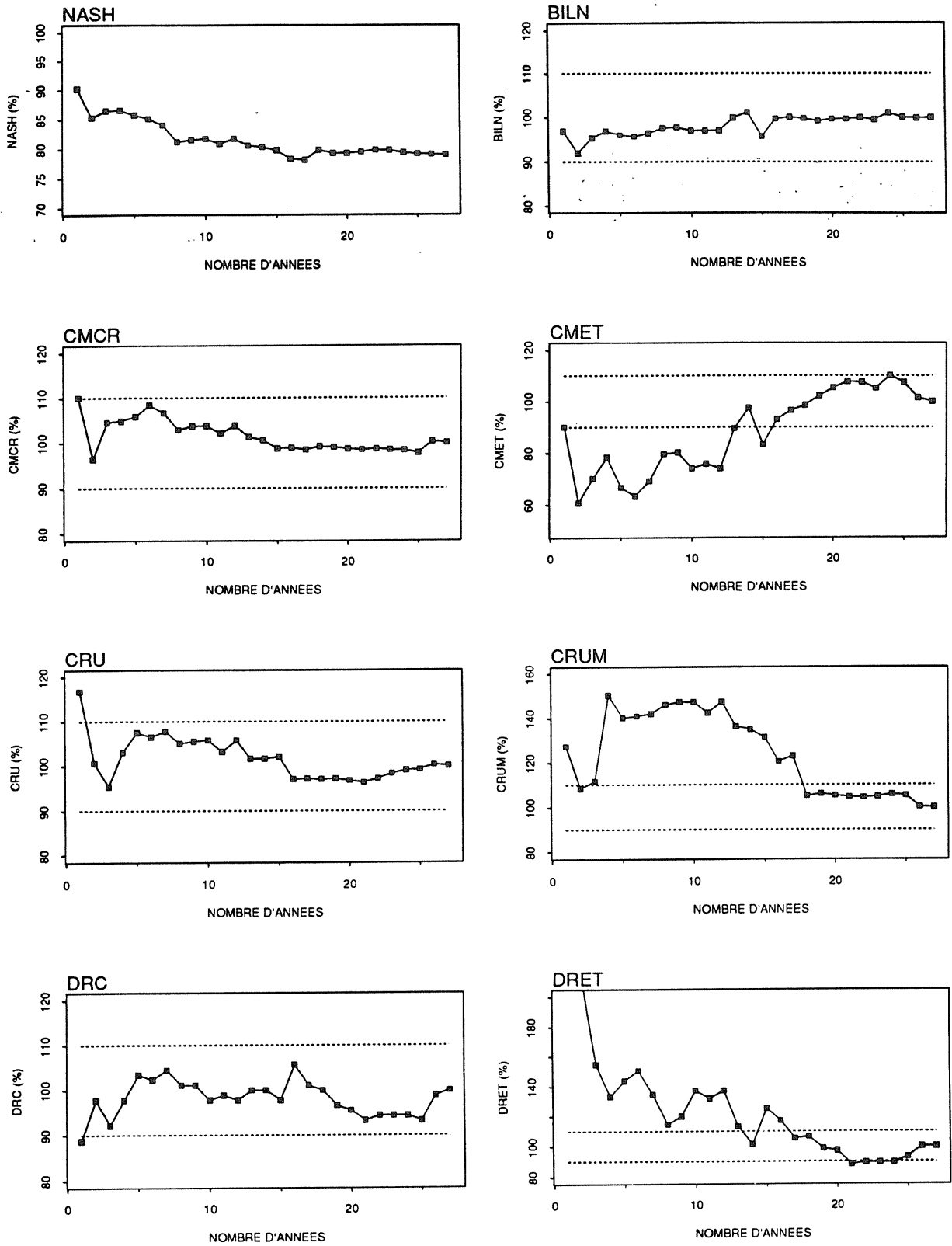
Fig. 4.11 - Bassin Versant de l'Orgeval - Evolution dans le temps des critères de qualité de GR4J en calage - paramètres a , b , c et d - calés sur des périodes de longueur \sum_{t=0}^{t=26} t + 1
