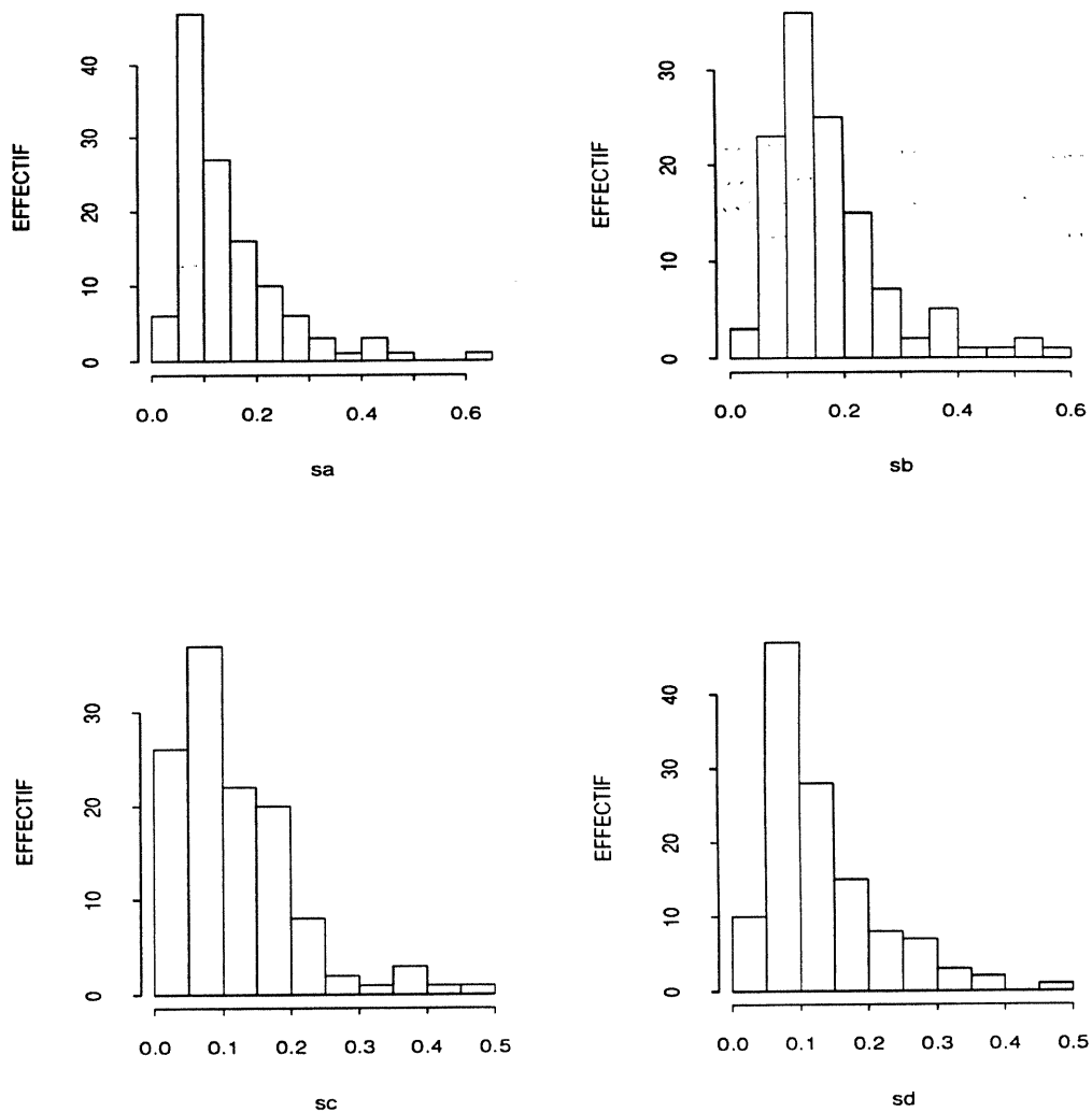
Fig. 3.11 - Sensibilité des paramètres pour 121 bassins versants
