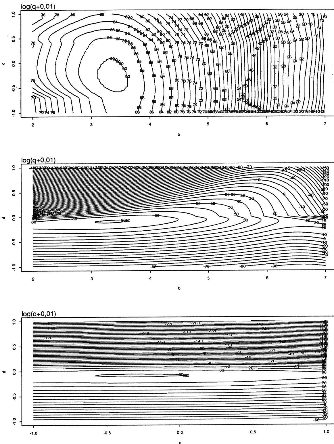
Fig. 5.39 - Méthode EG appliquée au modèle GR4J - courbes d'isocritere paramètres a-b, a-c, a-d, b-c; b-d et c-d - critère de NASH-T (transformation logarithmique) Bassin versant de l'Orgeval pour la période 1978-1980
