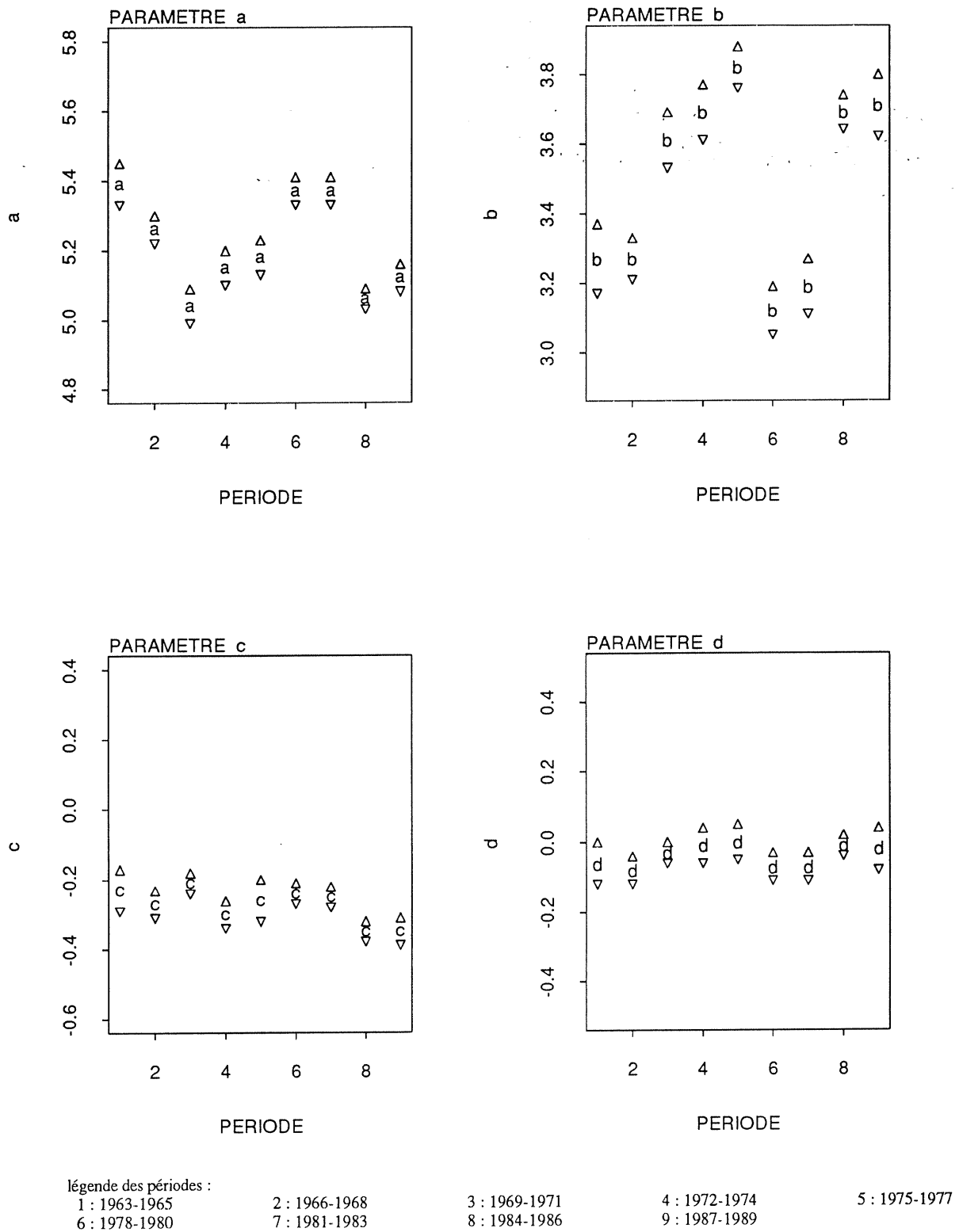
Fig. 6.6 - Paramètres a , b , c et d - calage de la série synthétique avec erreurs aléatoires ( k = 0,2 ) sur les pluies et les débits - 1963-1989, par période de 3 ans
