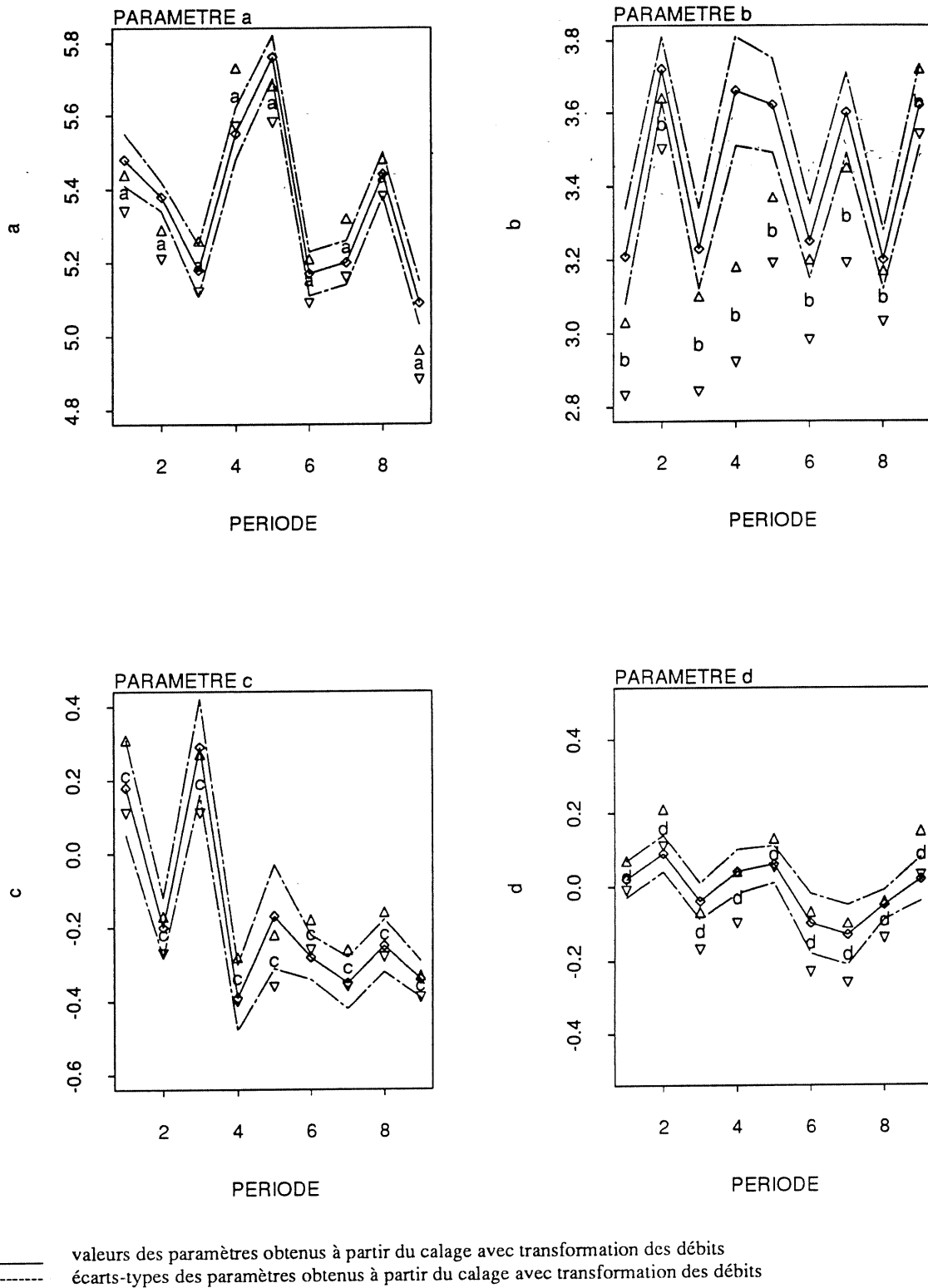
Fig. 5.25 - Bassin versant de l'Orgeval - paramètres a , b , c et d calage de GR4J sur la série 1963-1989 par période de 3 ans avec transformation des débits ( \lambda_1 = 0,5 )
