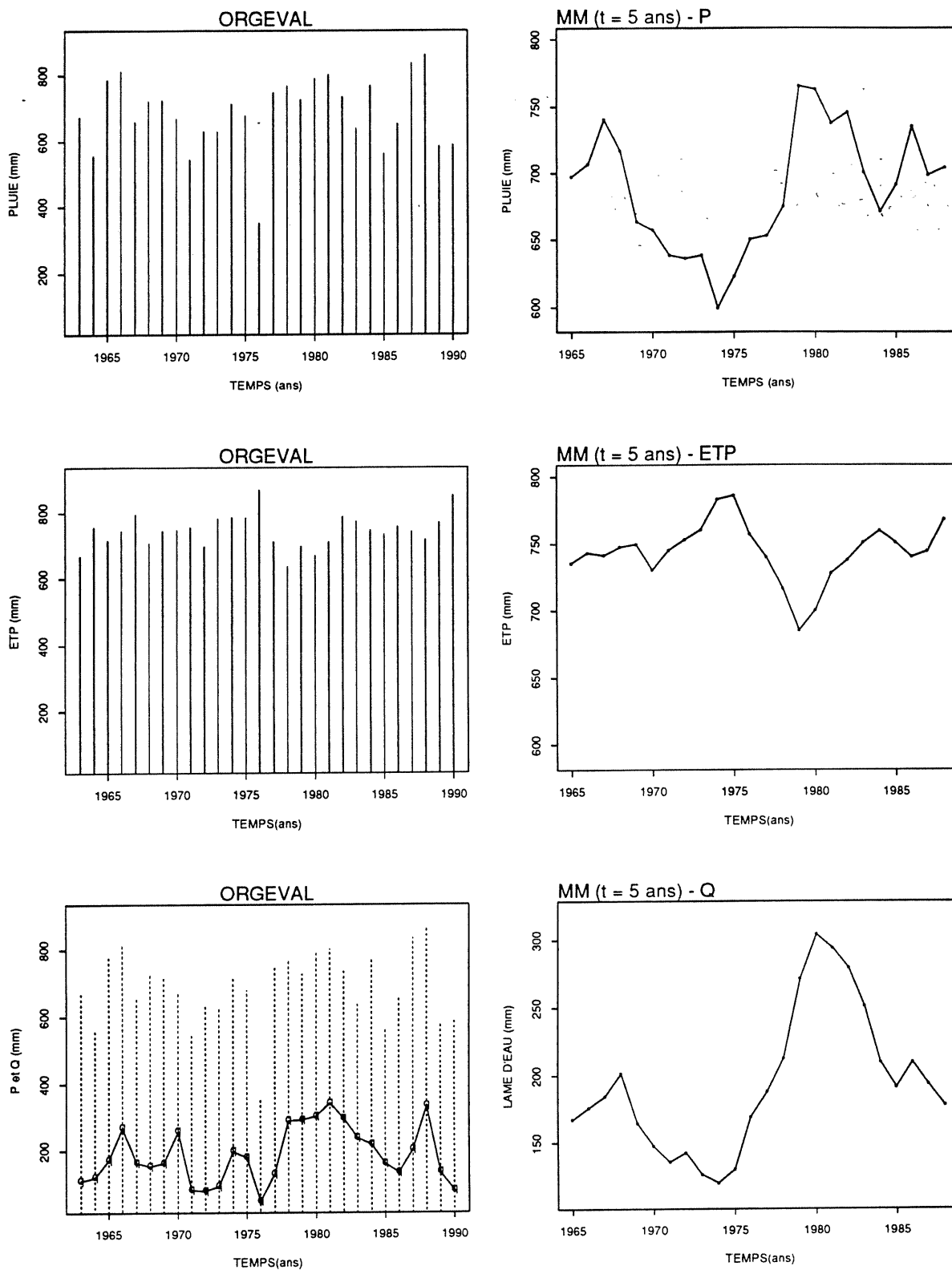
Fig. 4.2 - Bassin versant de l'Orgeval - précipitations, évapotranspiration potentielle et lames d'eau annuelles et ses moyennes mobiles (t = 5 ans)
