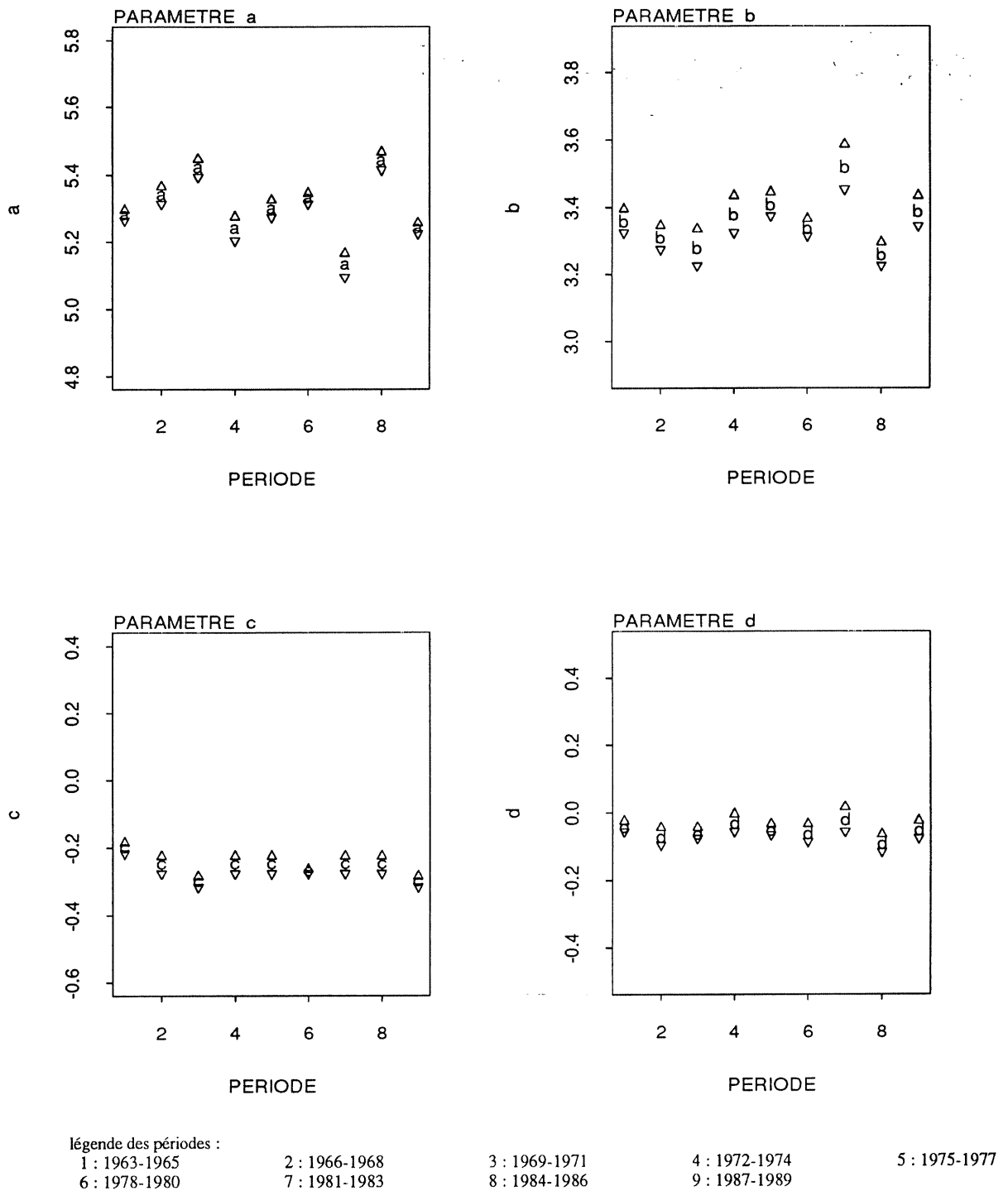
Fig. 6.5 - Bassin versant de l'Orgeval - paramètres a , b , c et d - calage de la série synthétique avec erreurs aléatoires ( k = 0,2 ) sur les débits - 1963-1989, par période de 3 ans
