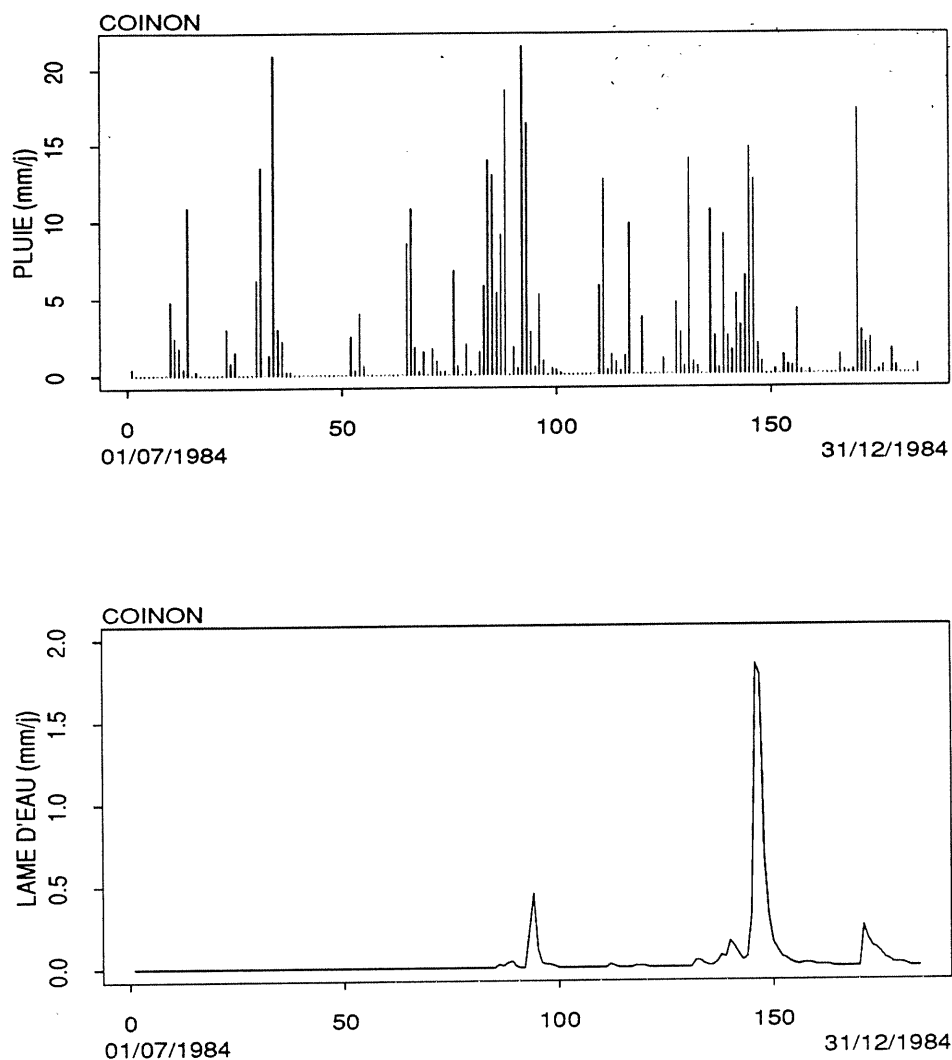
Fig. 2.5 - Hydrogramme d'un cours d'eau intermittent.
