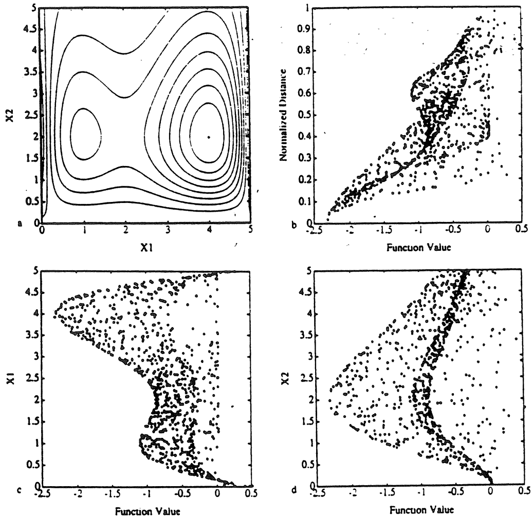
Fig. 5.1 - Méthode URS appliquée à la fonction d'Hosaki (a) courbes d'isocritères ; (b) distances réduites - fonction d'Hosaki ; (c) paramètre X_1 - fonction d'Hosaki ; (d) paramètre X_2 - fonction d'Hosaki. (d'après DUAN, SOROOSHIAN et GUPTA, 1992)
