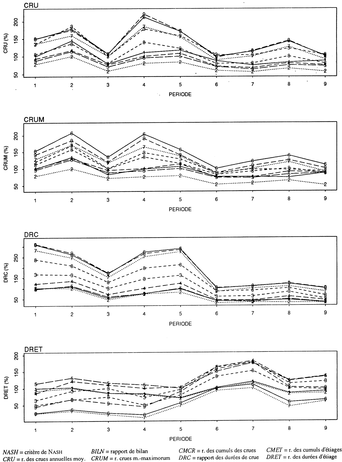
Fig. 6.19 - Evolution dans le temps des critères de qualité de GR4J pour des contrôles successifs (série synthétique [br.qtl100])
