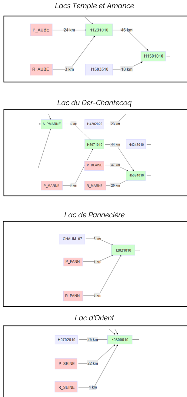
Figure 25 : Schématisation du réseau de stations hydrologiques du bassin de la Seine avec ajout des prises et restitutions de chaque lac-réservoir.
