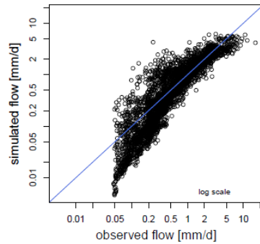
(d) SAC-SMA of sacsmAR.
